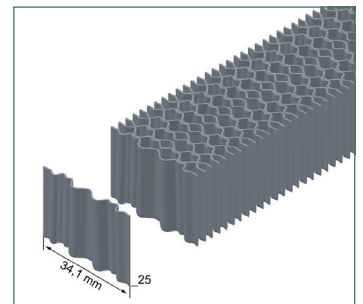
Abmessungen
